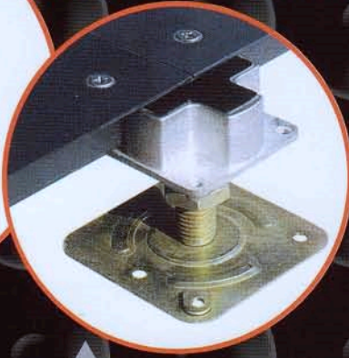
▲ Cornerlock
